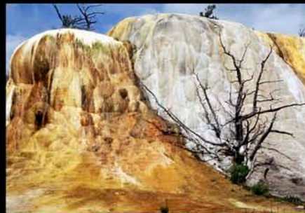
Kleurrijke kalk formaties, Yellowstone supervulkaan, USA, 2005
